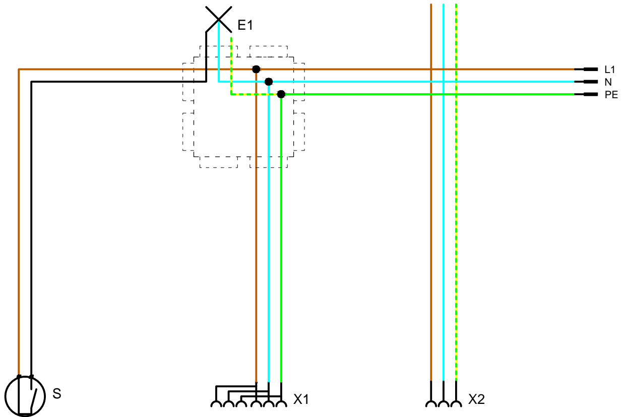
Bedradingschema
